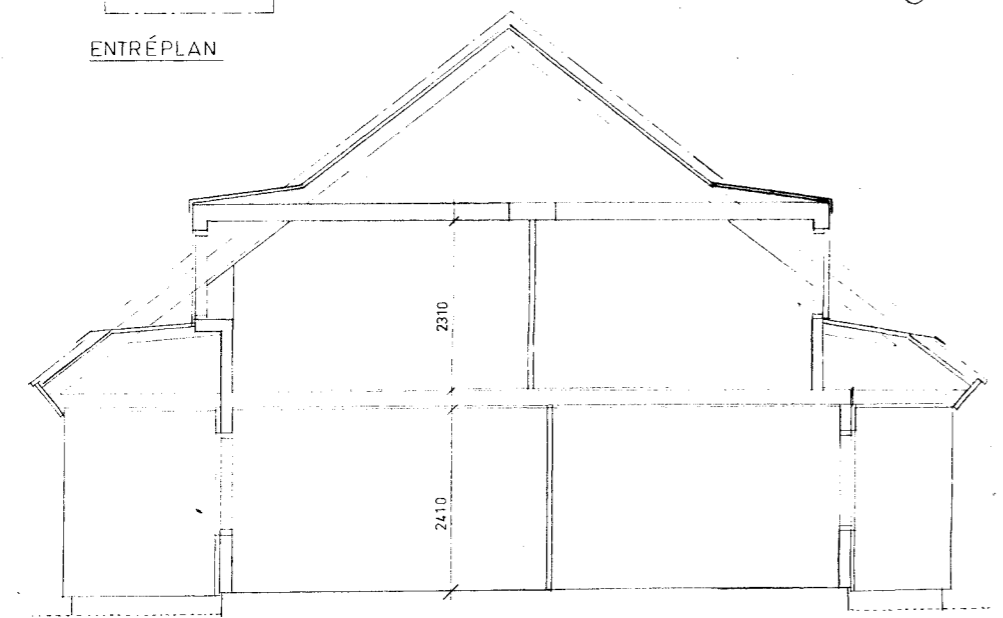
SEKTION
